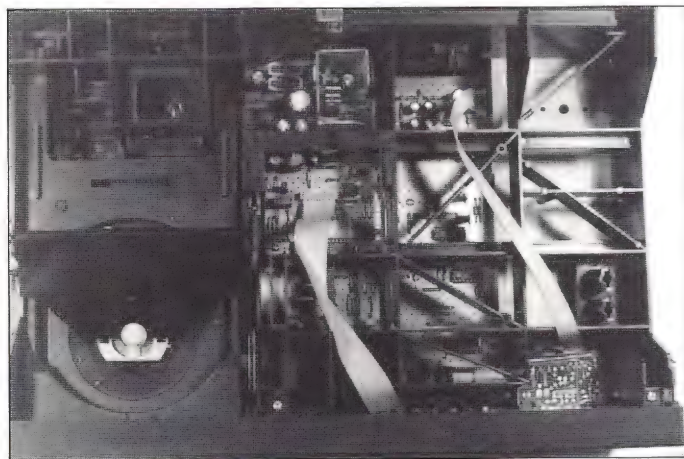
het inwendige van de Marantz speler met de kunststof versterkingsconstructie om de stijfheid van de kast te vergroten
